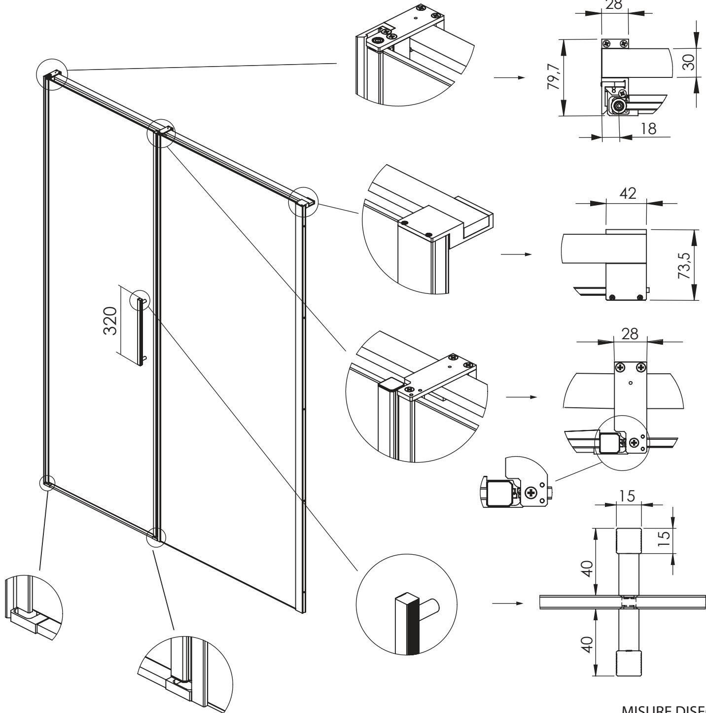
MISURE DISEGNO TUTTE IN MM
